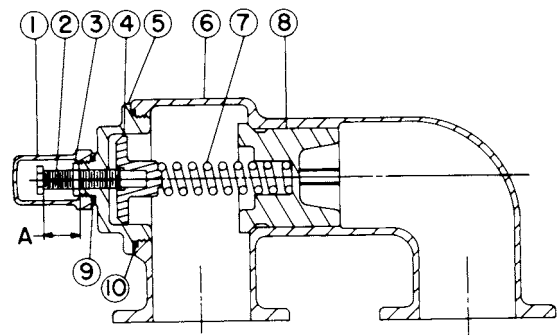
VENTIL - TEILELISTE
