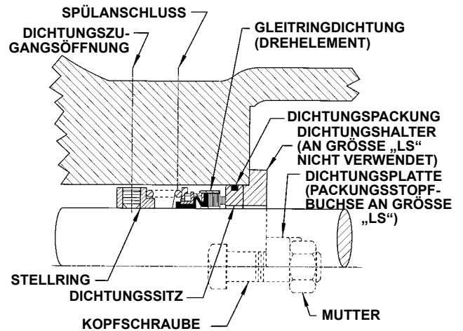
ABBILDUNG 9 ELASTOMER-FALTENBALG-DICHTUNG
