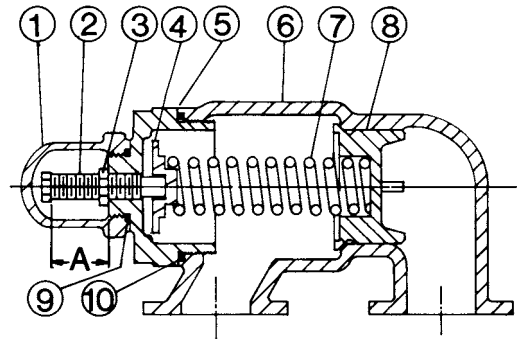
VENTIL - TEILELISTE
